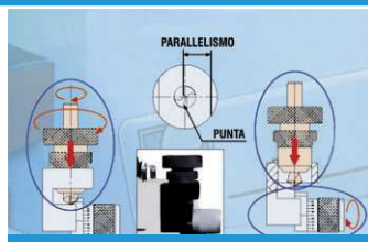
Regolazione della lunghezza e posizionamento della punta
