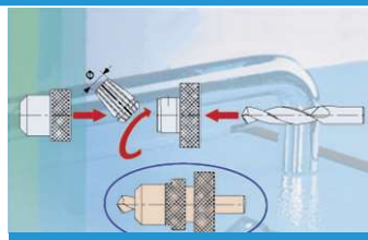
Preparazione della punta per l'affilatura
